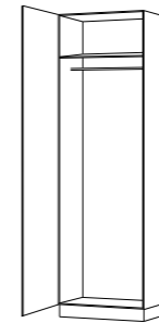
1x Hyllplan Fast 1x Klädstång BREDD: 400 - 800 MM
