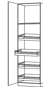
1x Hyllplan Fast 4x Invändig låda BREDD: 600 MM
