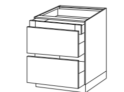
2x Grytlåda & 1x Invändig låda BREDD: 300 – 1000 MM
